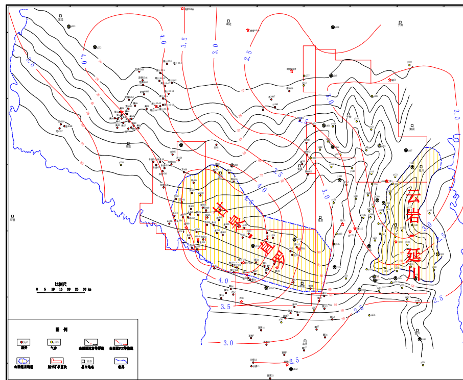
延长页岩气勘探有利区综合评价图
