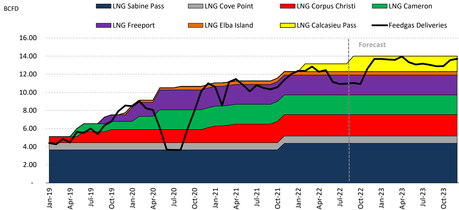
U.S. LNG Export Capacity vs. Feedgas Deliveries
